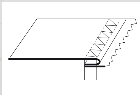
DIBUJO TÉCNICO
